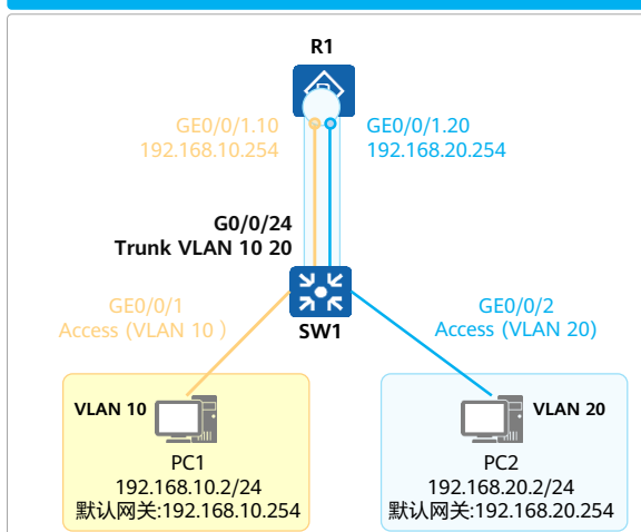
物理连接图
