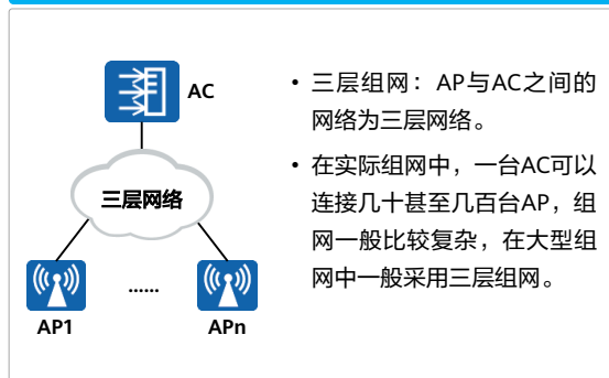
三层组网
