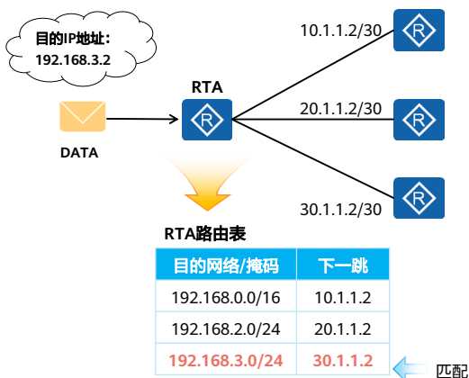
最长匹配示例
