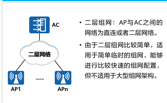
二层组网
