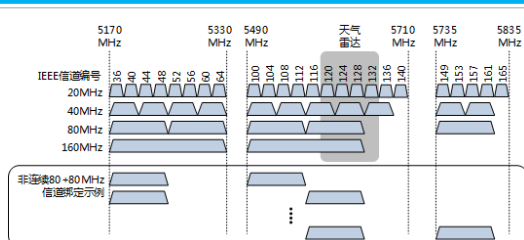
5GHz频段
